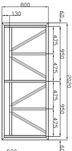
VISTA INFERIOR
